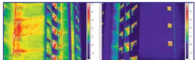
Thermographieaufnahmen vor und nach der Sanierung
